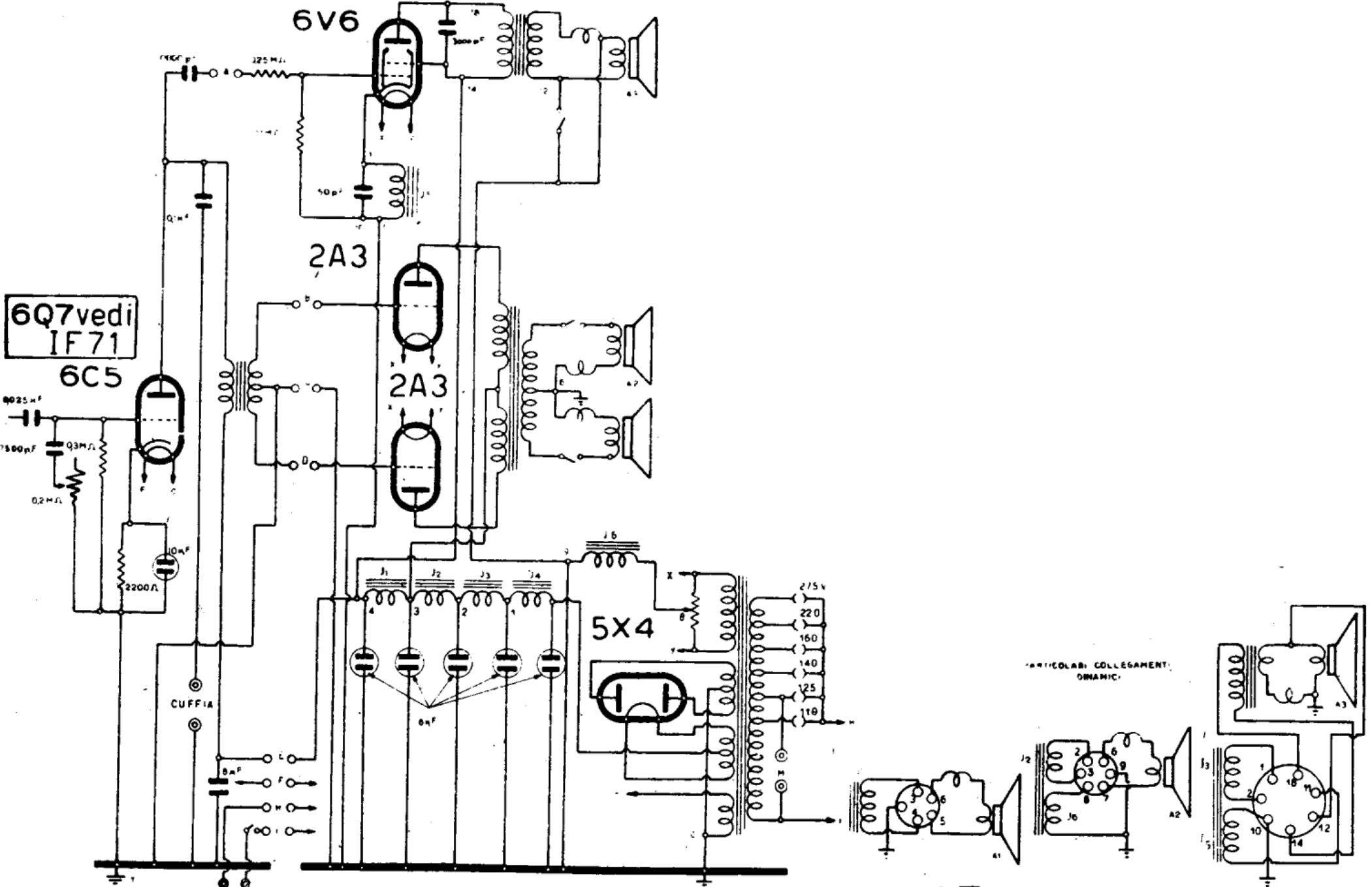
Questi due circuiti si accordano con il modello « IF 71 » III serie di cui è stato riprodotto lo schema
